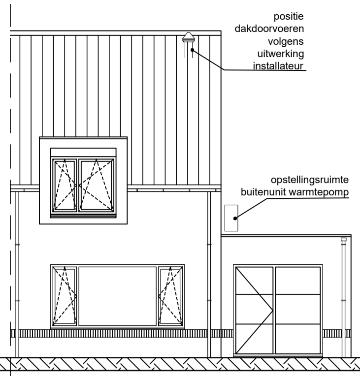
Voorgevel
