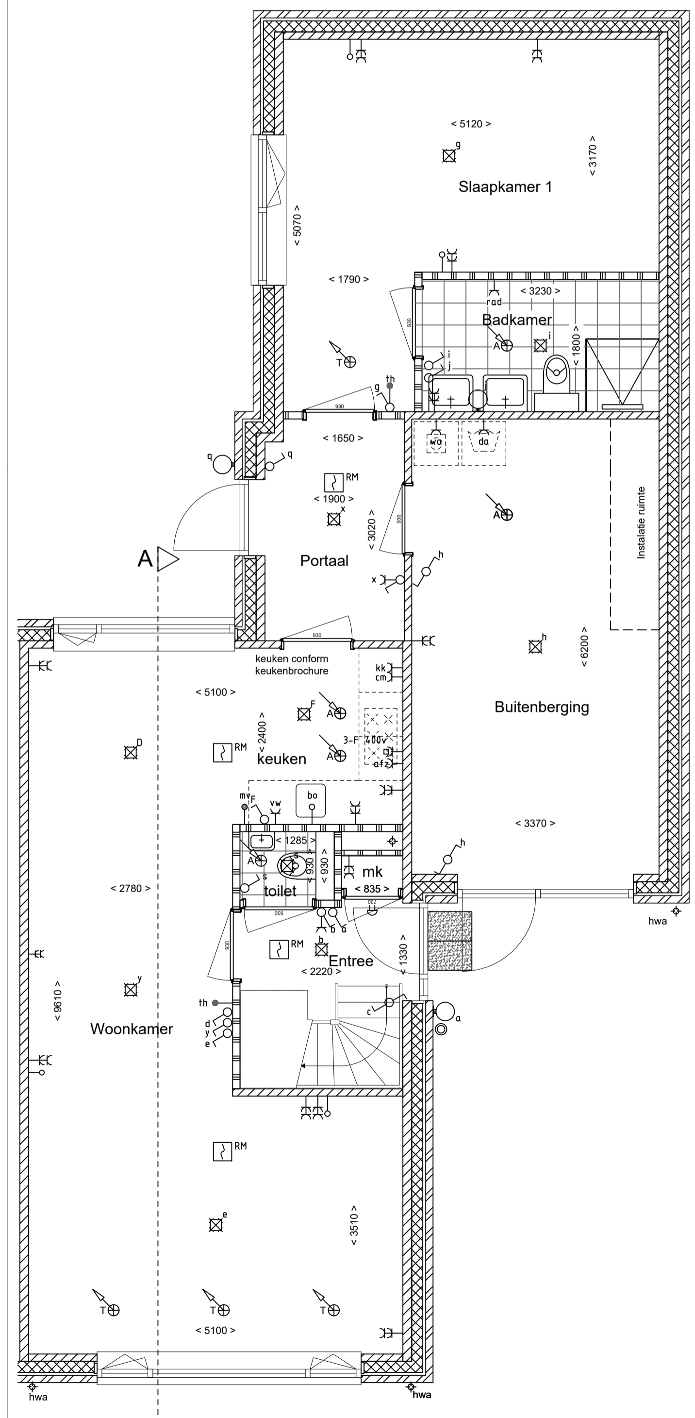
Begane grond
