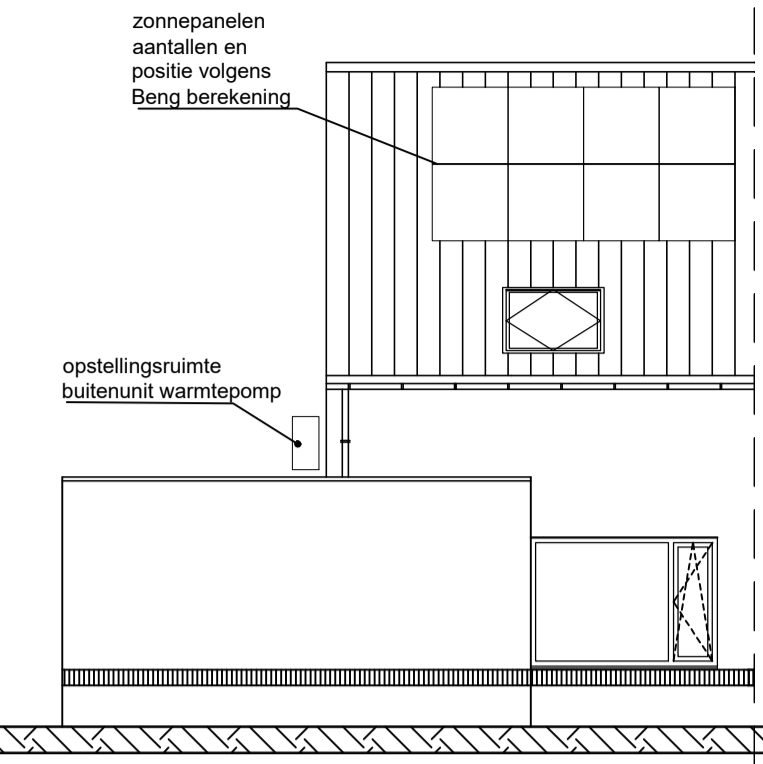
Achtergevel
